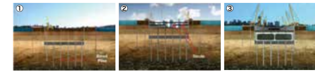
①陸化を終え、トンネル函体を支える底盤を地盤改良し、その基礎になる杭を打設する ②陸化を終えた部分は、軟弱地盤のため沈下の恐れが小さい小型の掘削機械を用いて、切梁を設置しながら掘り進めていく ③掘削を終え、トンネル函体を構築し終えたところ。天端には厚さ1mほどの保護コンクリートを打設したうえで土砂を埋め戻す
